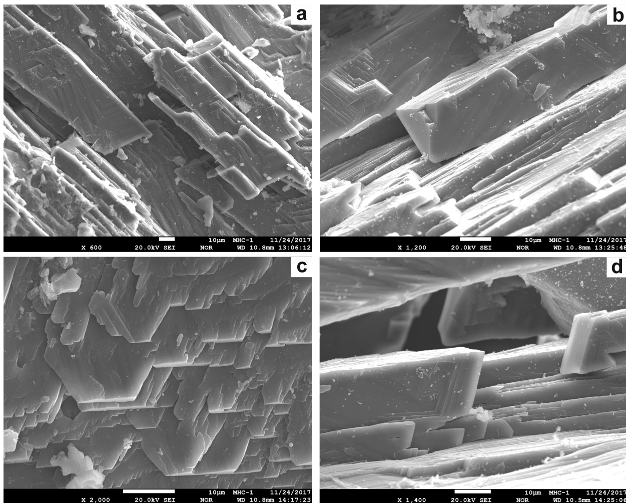
Obr. 3 (a - d) Stĺpcovité a ihlicovité kryštály MHC tvoriace paralelné zrazy jednotlivých kryštálov. SEM foto T. Mikuš.
