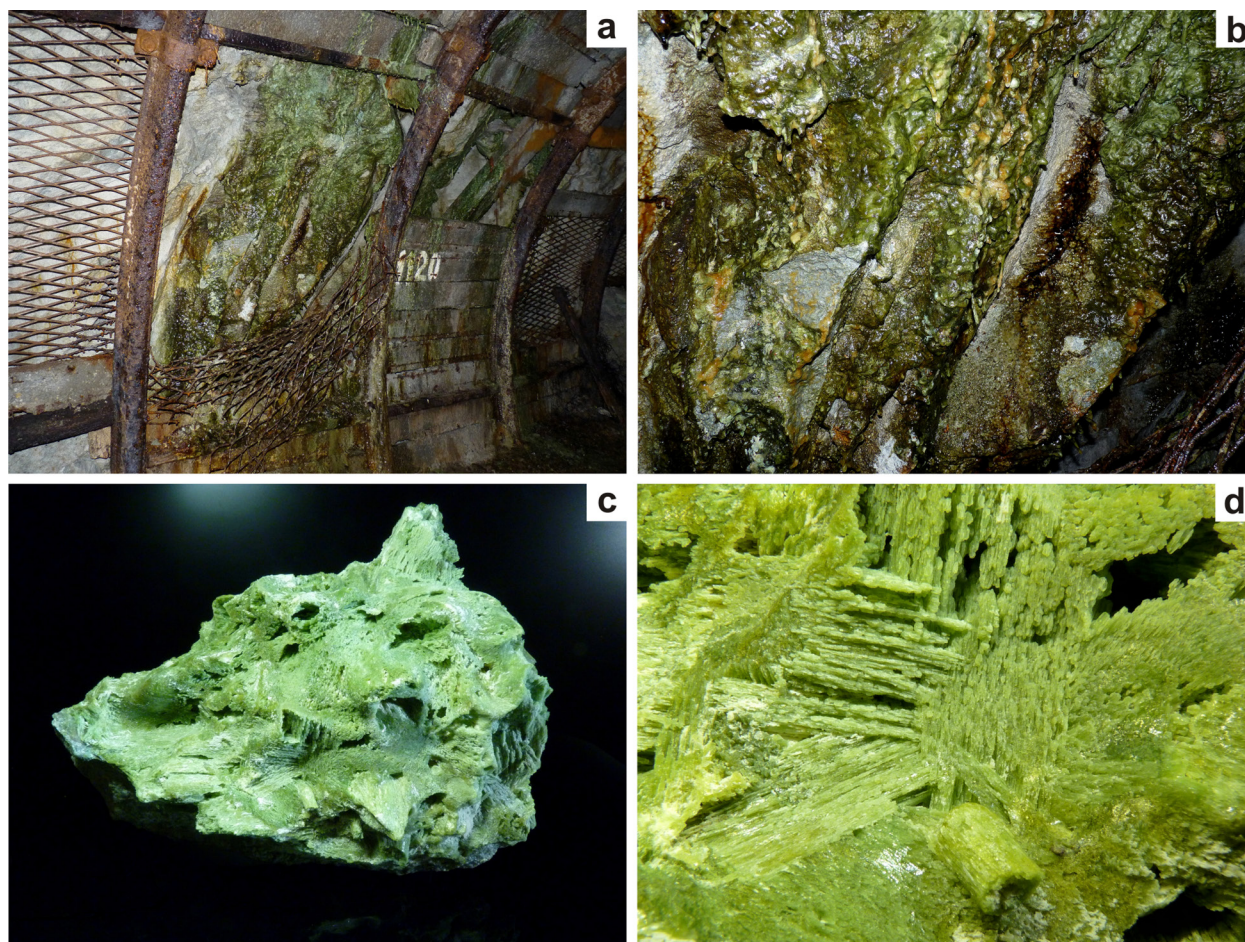
Obr. 2 a) Miesto výskytu sekundárnych karbonátov v Piesockej štôlni, plocha na ktorej sa vyskytuje monohydrokalcit má 100 \times 80\text{ cm} ; b) detailný záber na náteky pripomínajúce jaskynný sinter, veľkosť záberu 30 \times 40\text{ cm} ; c) masívny agregát monohydrokalcitu, veľkosť vzorky 15 \times 10\text{ cm} ; d) kryštalický agregát monohydrokalcitu, šírka záberu 15 \times 20\text{ mm} . Foto T. Bancík.
