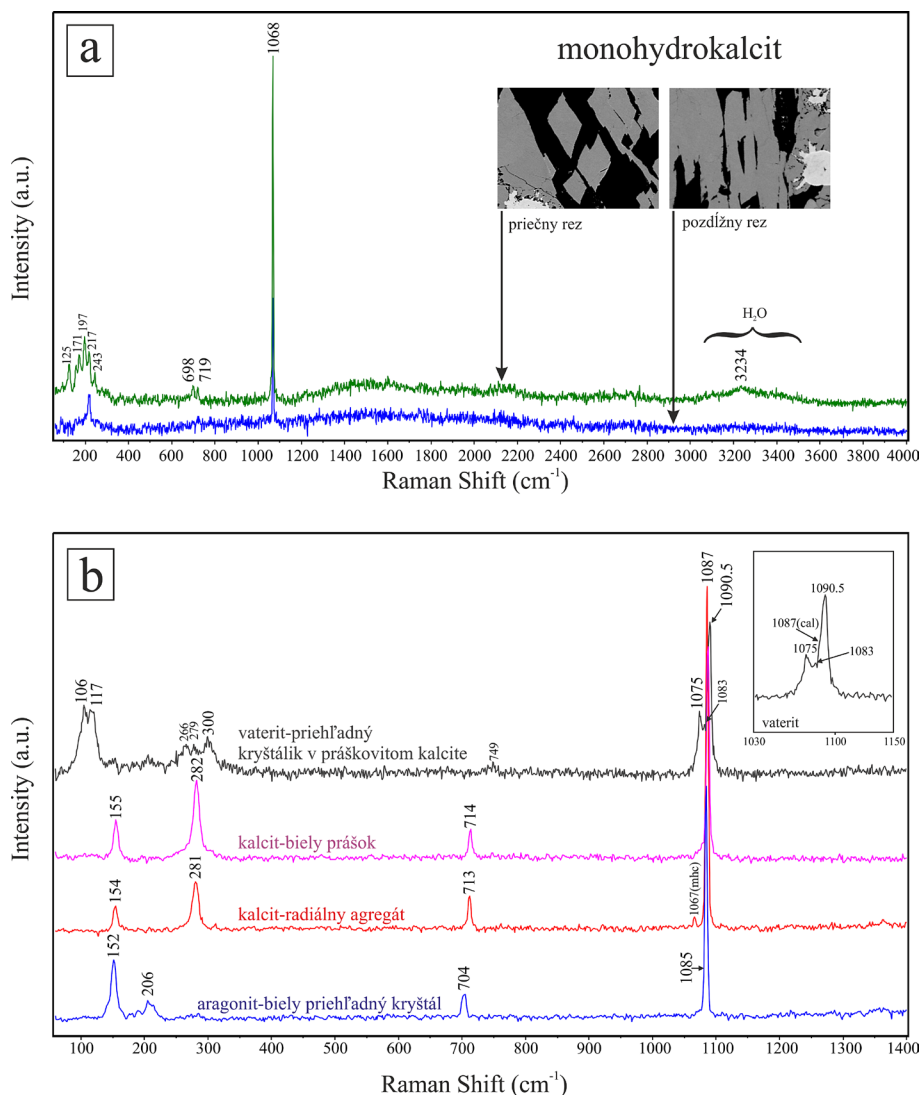
Obr. 7 Ramanove spektrá sekundárnych karbonátov Ca zo Španej Doliny. a) Ramanove spektrá monohydrokalcitu nasnímané z rôzne orientovaných kryštálov - pričný a pozdlžný rez, v spektre priečného rezu kryštálu sú viditeľné vibrácie vody; b) Ramanove spektrá rôznych fáz \text{CaCO}_3 zistených v asociácii s monohydrokalcitom. Vložený obrázok detailne znázorňuje Ramanove pásy iónu \text{CO}_3^{2-} vo vaterite. Skratky: cal - kalcit; MHC - monohydrokalcit.
